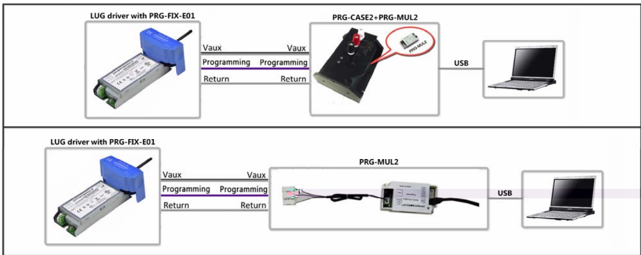
PRG-FIX-E01 LUG
