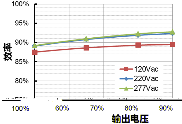
EUP-240S150ST (Io=1500mA) 效率 vs. 输出电压
